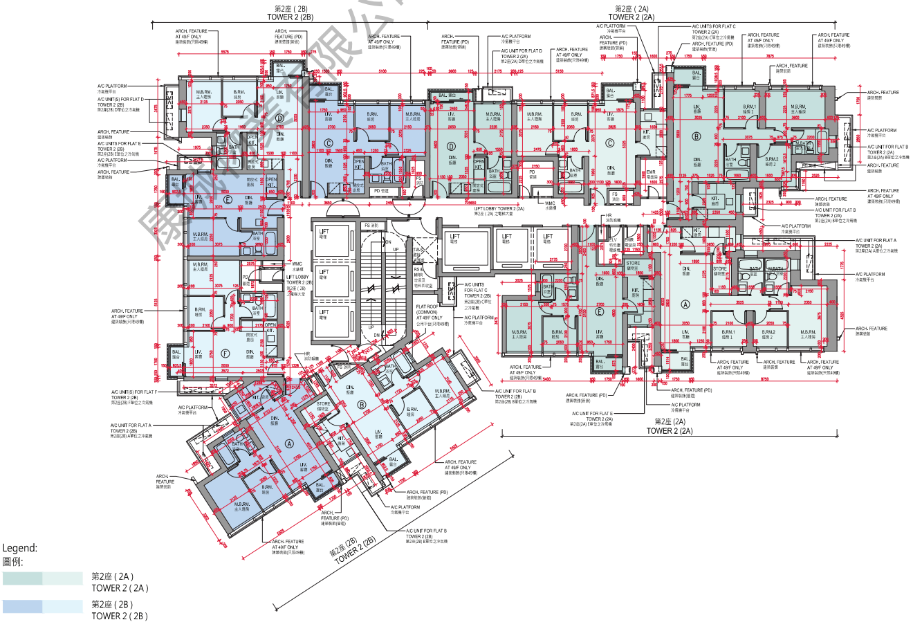
TOWER 2 (2A & 2B) 49/F-53/F, 55/F-63/F AND 65/F-70/F FLOOR PLAN 第2座 (2A & 2B) 49樓至53樓、55樓至63樓及65樓至70樓樓面平面圖
